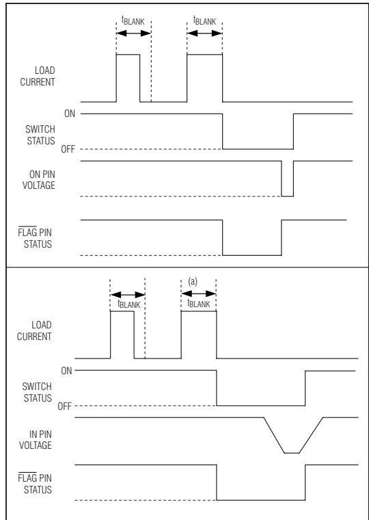
图 3. MAX4795/MAX4797 闭锁故障屏蔽
