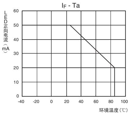
LED正向电流—环境温度
