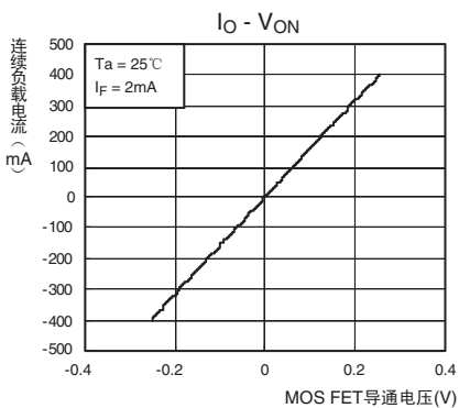
连续负载电流—MOS FET导通电压
